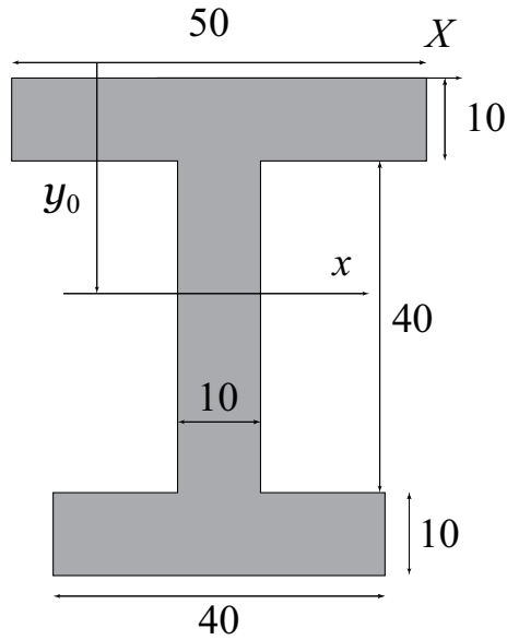
図 1: 上下非対称 I 型断面
